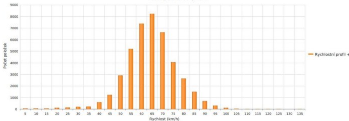
Býkovec, Směr od Kališ, 50 km/h povolená rychlost Počet položek vs. rychlost
